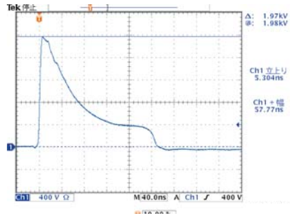
EUT LINE OUTPUT waveform : 50Ω
